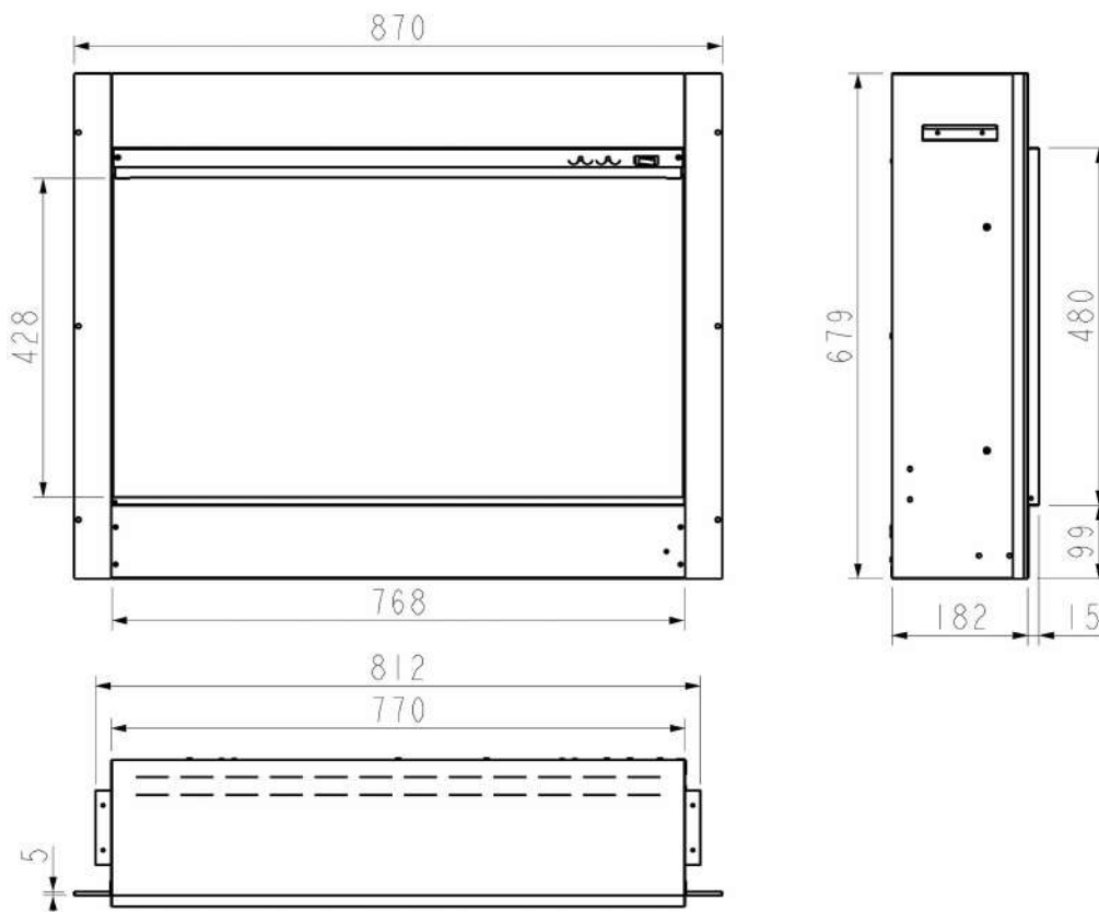
Fig. 1 - Fire Dimensions
